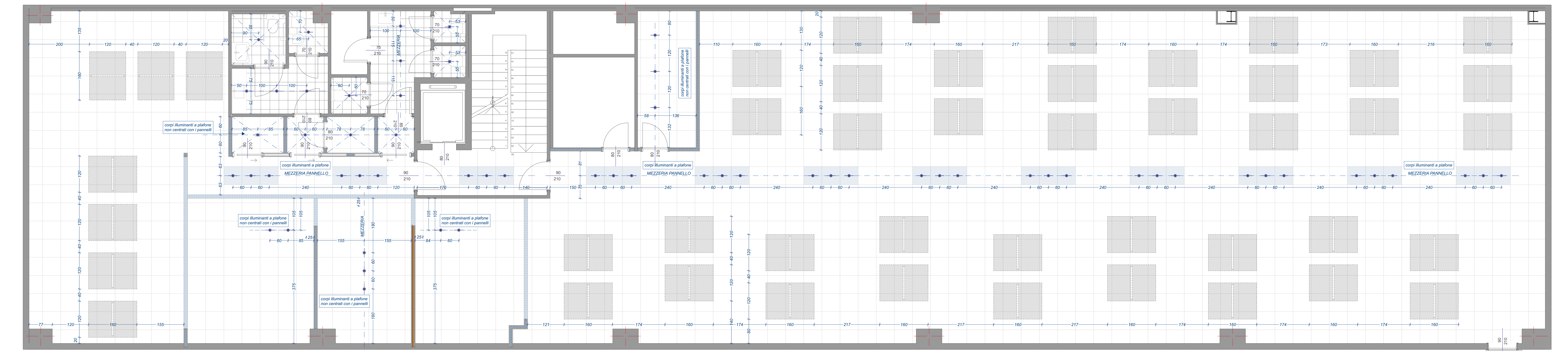
LAYOUT POSIZIONE PANNELLI ACUSTICI E CORPI ILLUMINANTI - ALLINEAMENTO CONTROSOFFITTO
